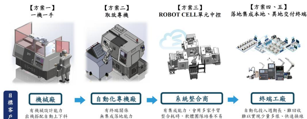
圖四、新代與聯達機器人解決方案
